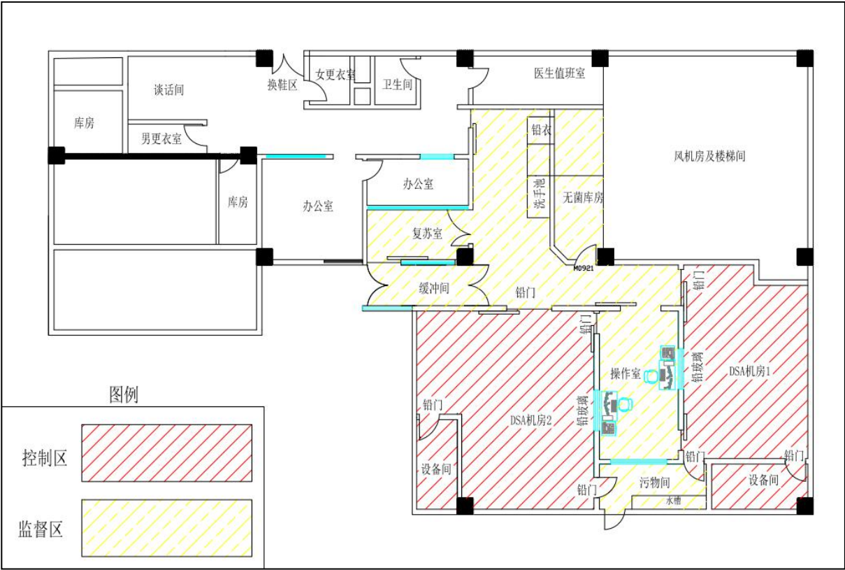
图 10-1 本项目 DSA 两区划分示意图
