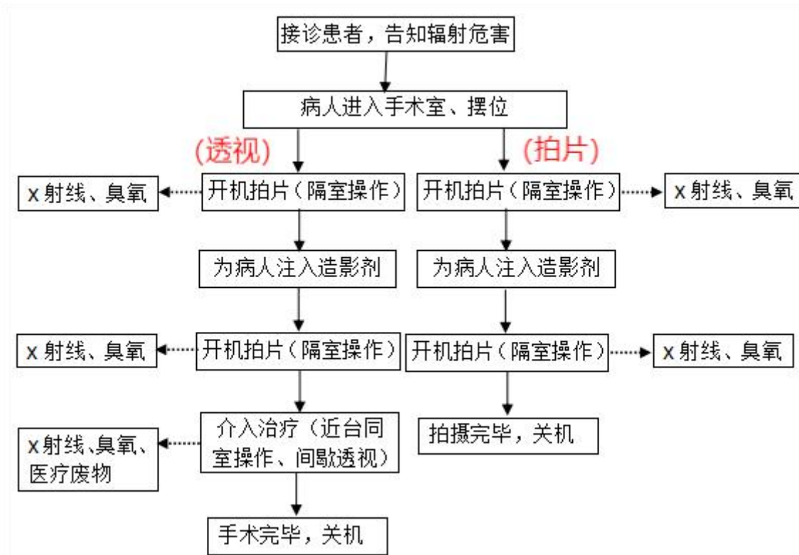
图 9-2 DSA 介入治疗流程及产污环节示意图
