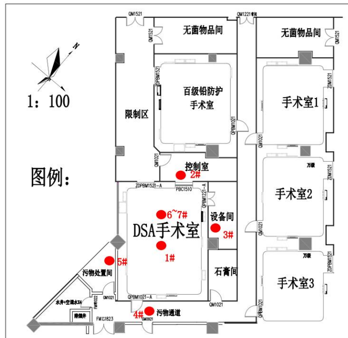
图8-2 本项目DSA手术室周围现状监测布点示意图
