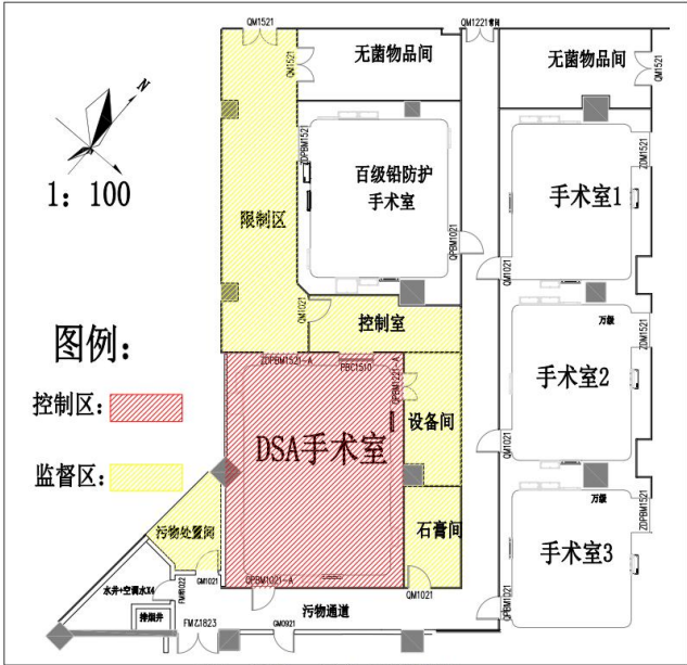
图 10-1 DSA 手术室两区划分示意图
