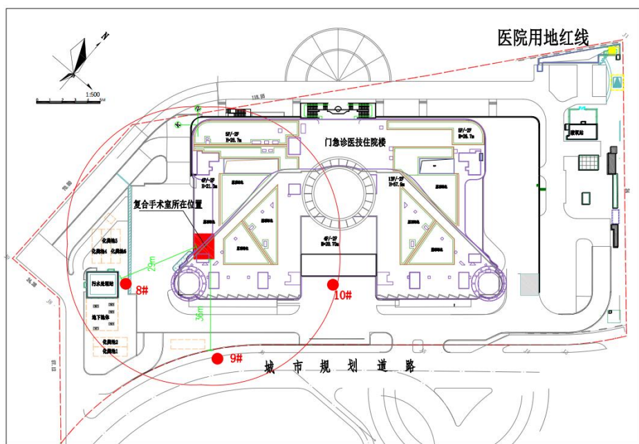
图8-2 本项目DSA手术室周围现状监测布点示意图
