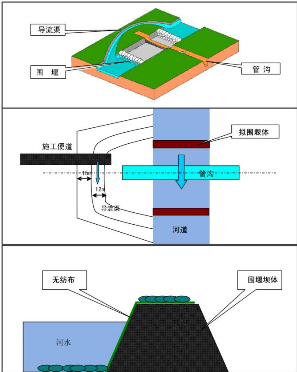
图 3-5 围堰导流开挖管沟法施工断面示意图
