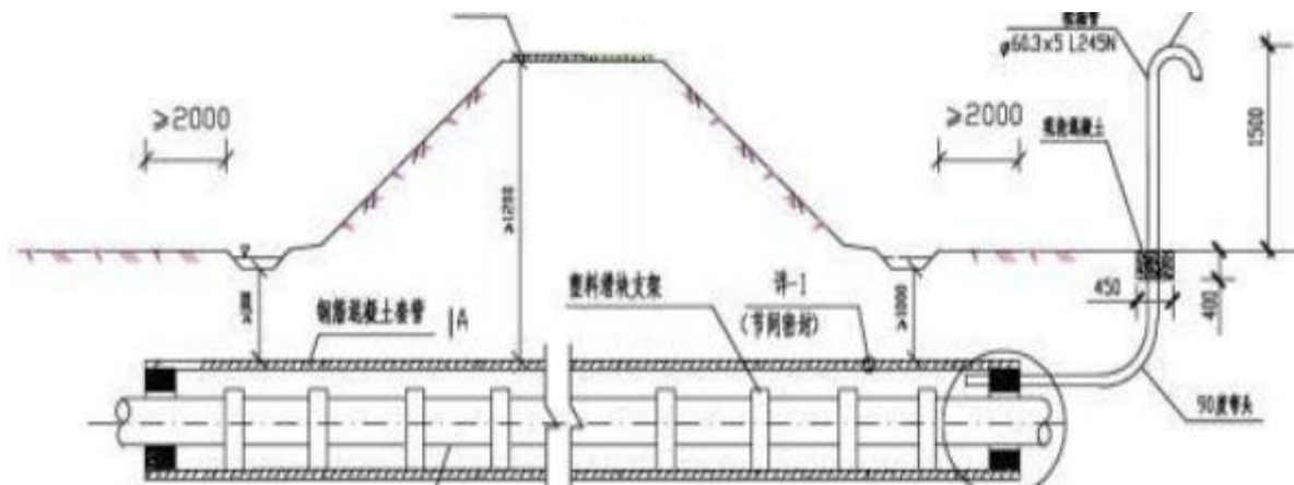
图 3-4 管道穿越乡村水泥路断面示意图
