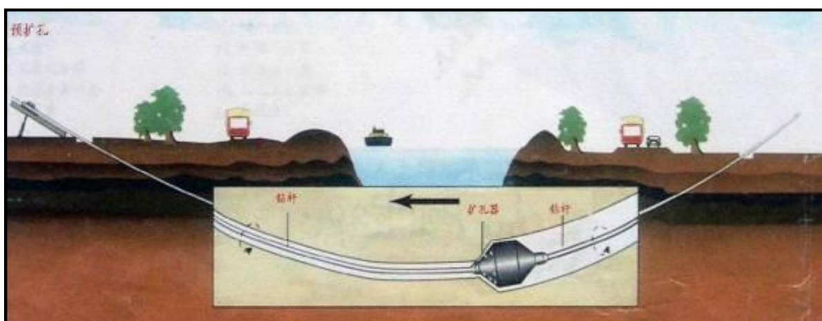
图 3-7 定向钻穿越施工预扩孔过程断面示意图
