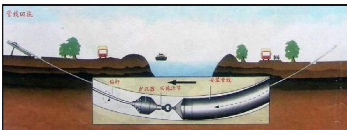
图 3-8 定向钻穿越施工管线回拖过程断面示意图
