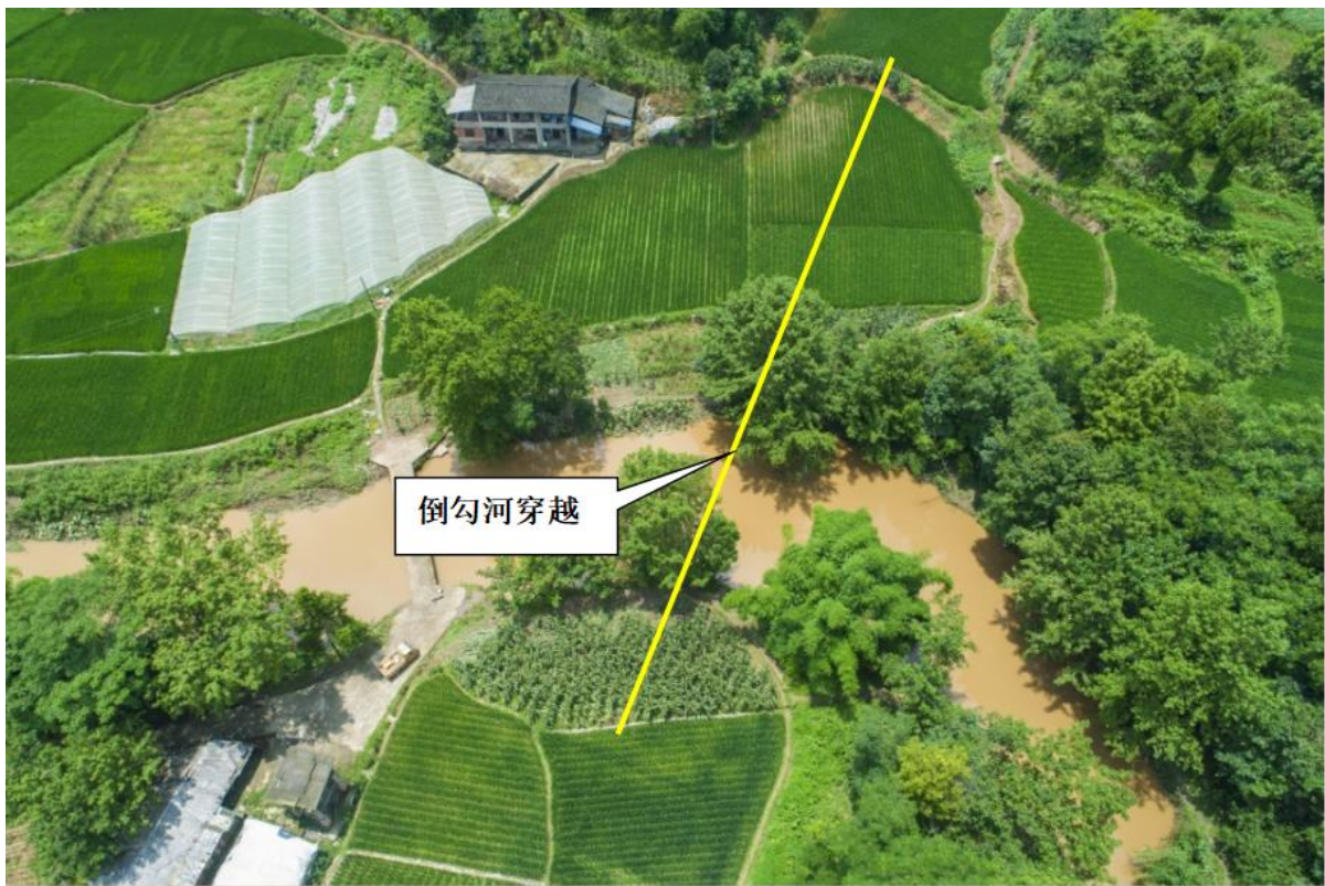
图 5-2 倒勾河定向钻穿越位置图
