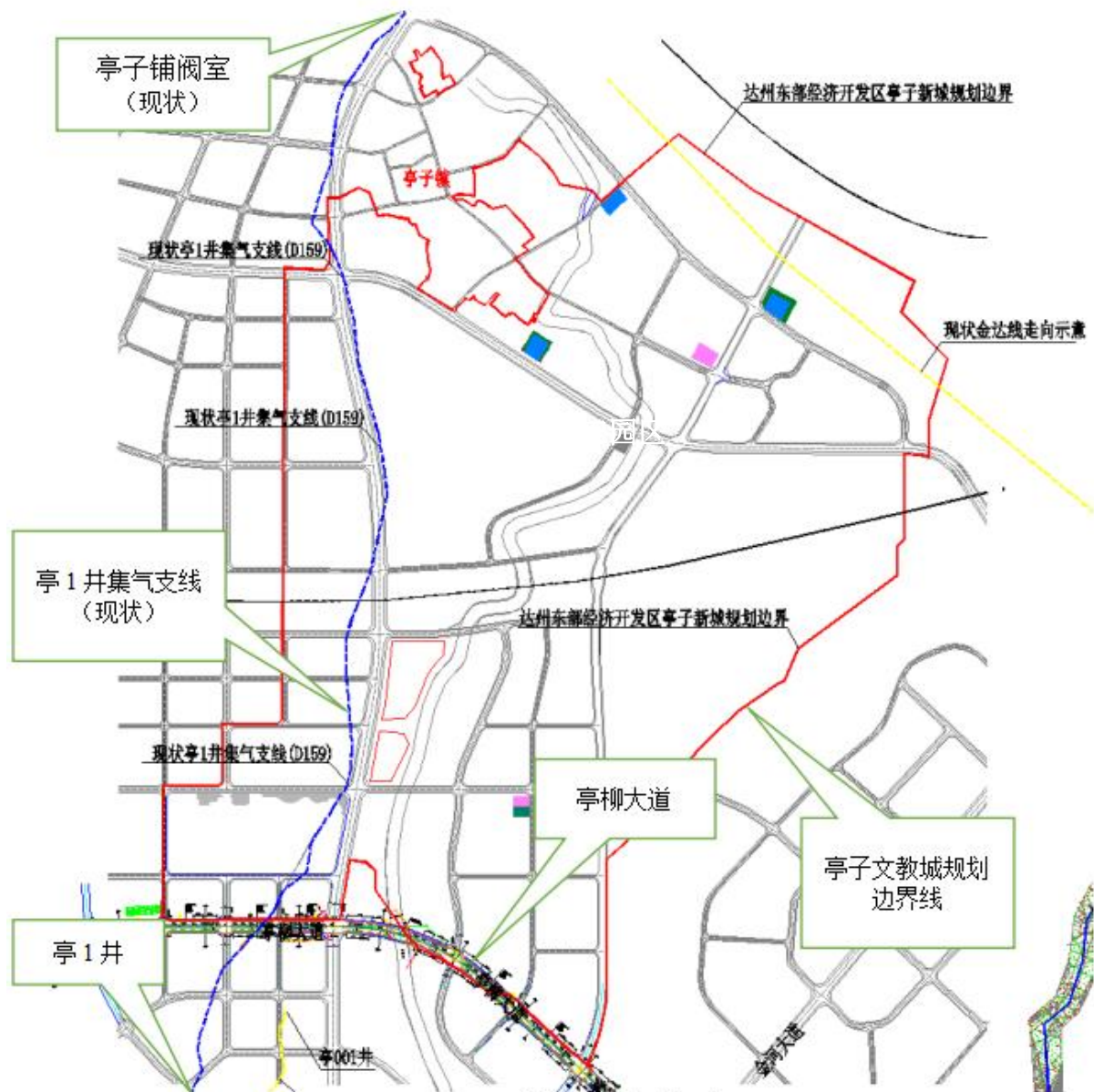
图 2-2 现状管线与规划区交叉
