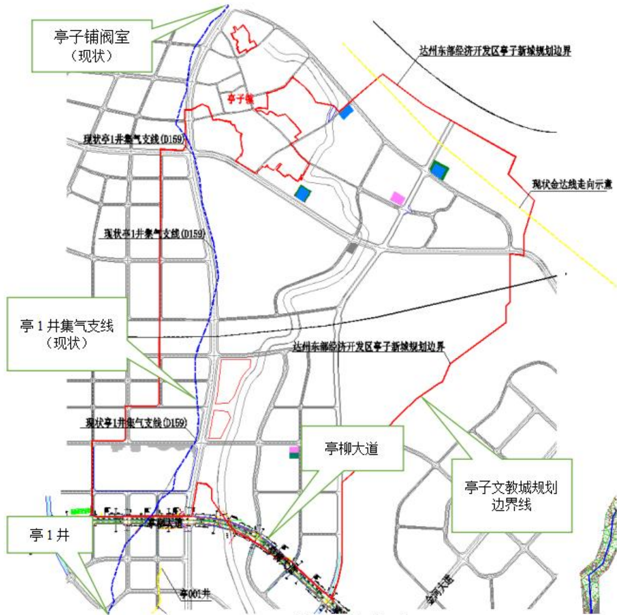
图 1-1 规划化工园区内现有集气管线分布图（蓝线表示）
