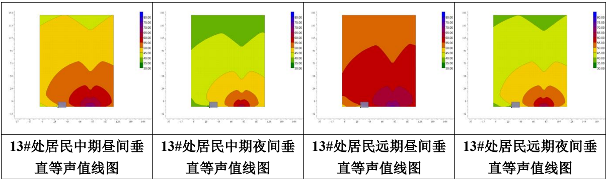
图 5.2-18 代表性敏感保护目标垂直断面等声级线图（绕场镇段）
