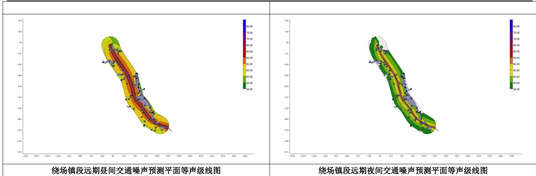
图 5.2-17 绕场镇段交通噪声预测平面等声级线图
