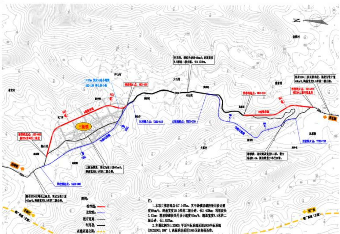
图 3.1-1 路线方案比较图
