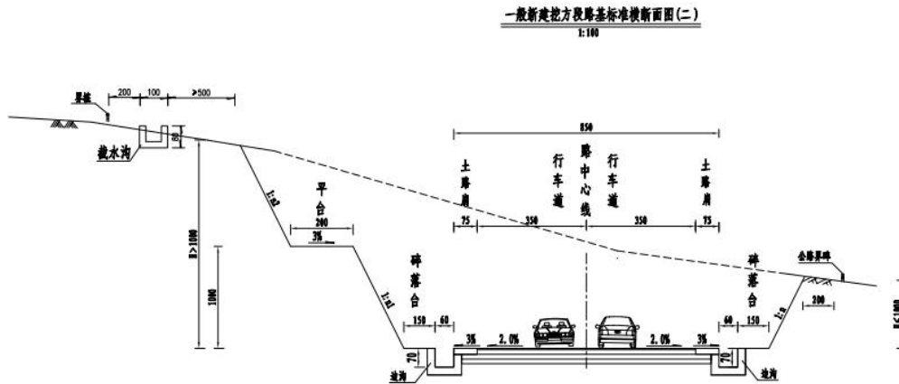
图 2.3-2 路基标准横断面图（绕地灾段）
