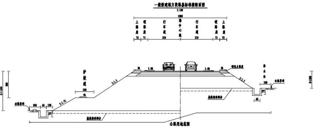
图 2.3-1 路基标准横断面图（绕场镇段）
