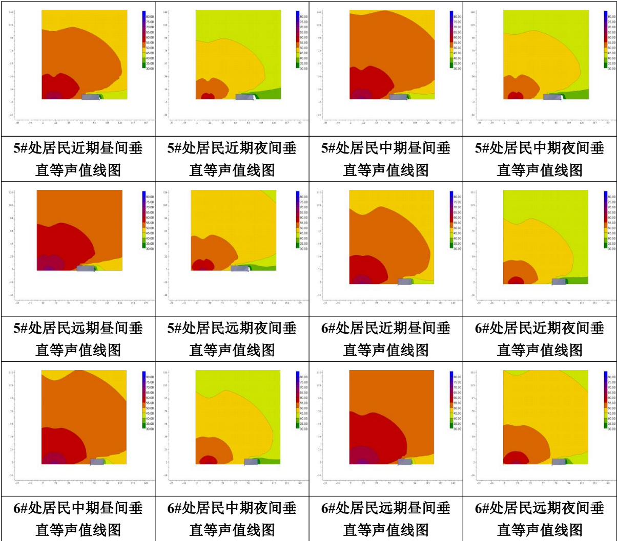
图 5.2-18 代表性敏感保护目标垂直断面等声级线图（绕地灾段）
