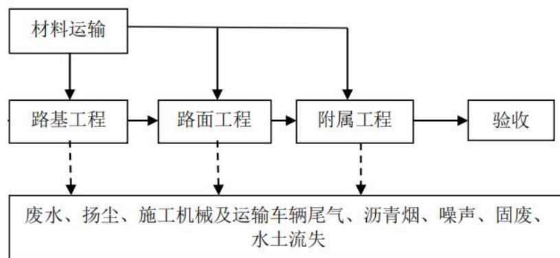
图 3.2-2 道路工程施工工艺流程及产污环节图
