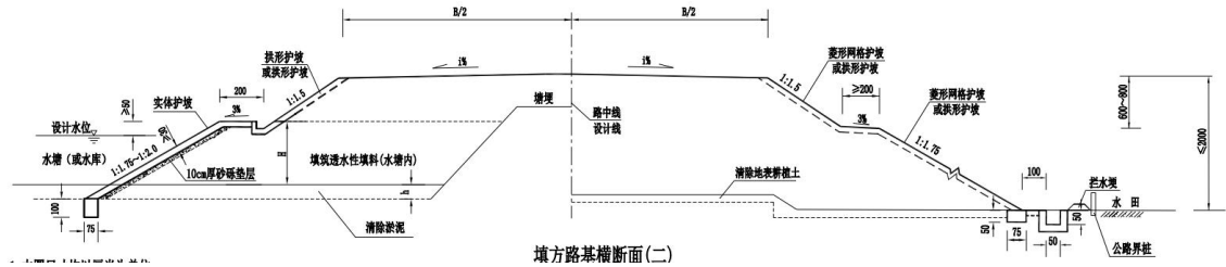
图 2.3-3 路基标准横断面图（填方路基）
