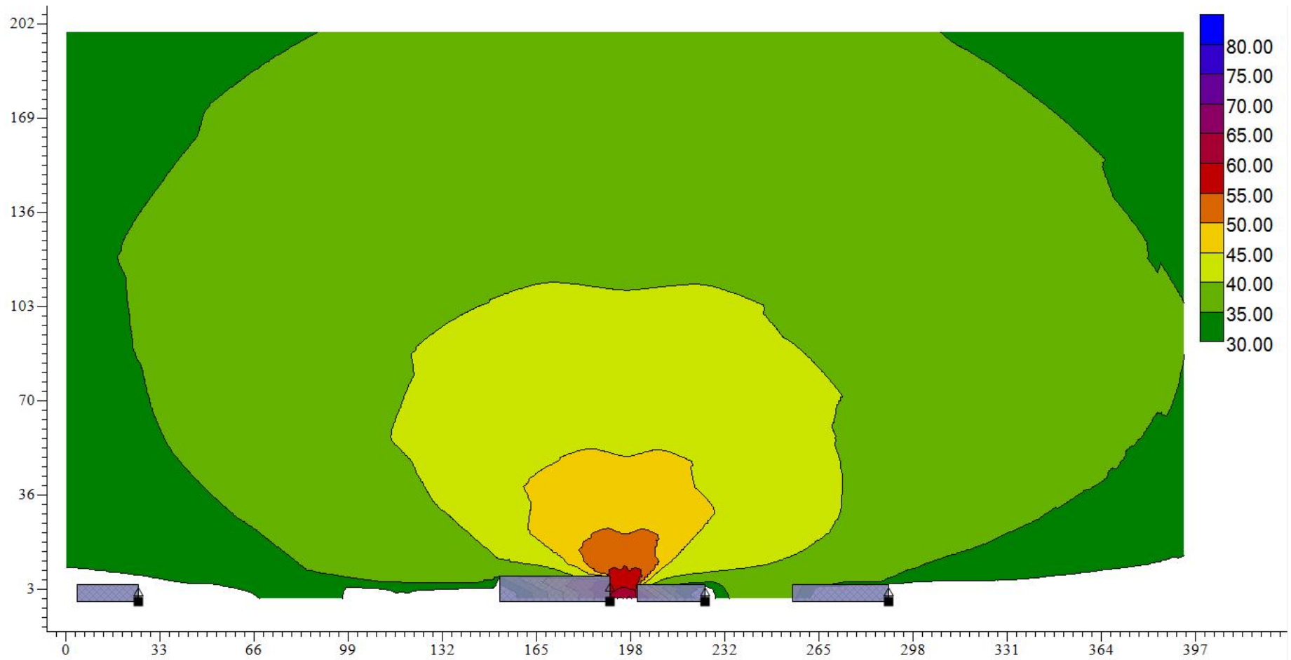
图 5.2-9.2 项目 K3+175.765 北侧 12m 农户处垂直等声值线图（近期夜间）
