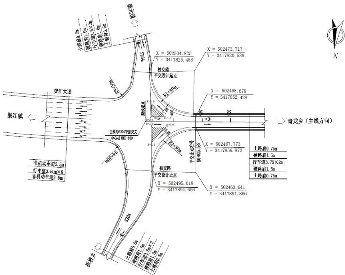
图 2.3-6 K0+000 平面交叉
