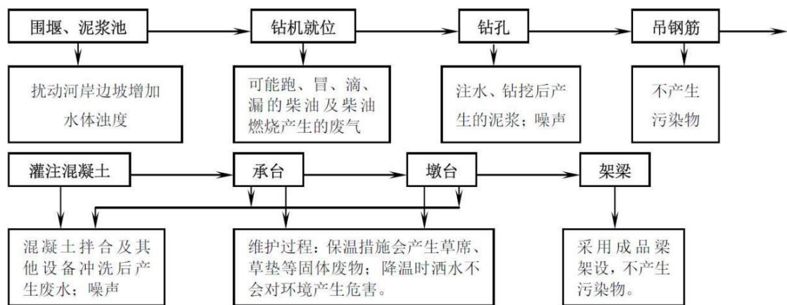
图 3.2-3 钻孔灌注桩基础施工工艺流程及环节产污情况图
