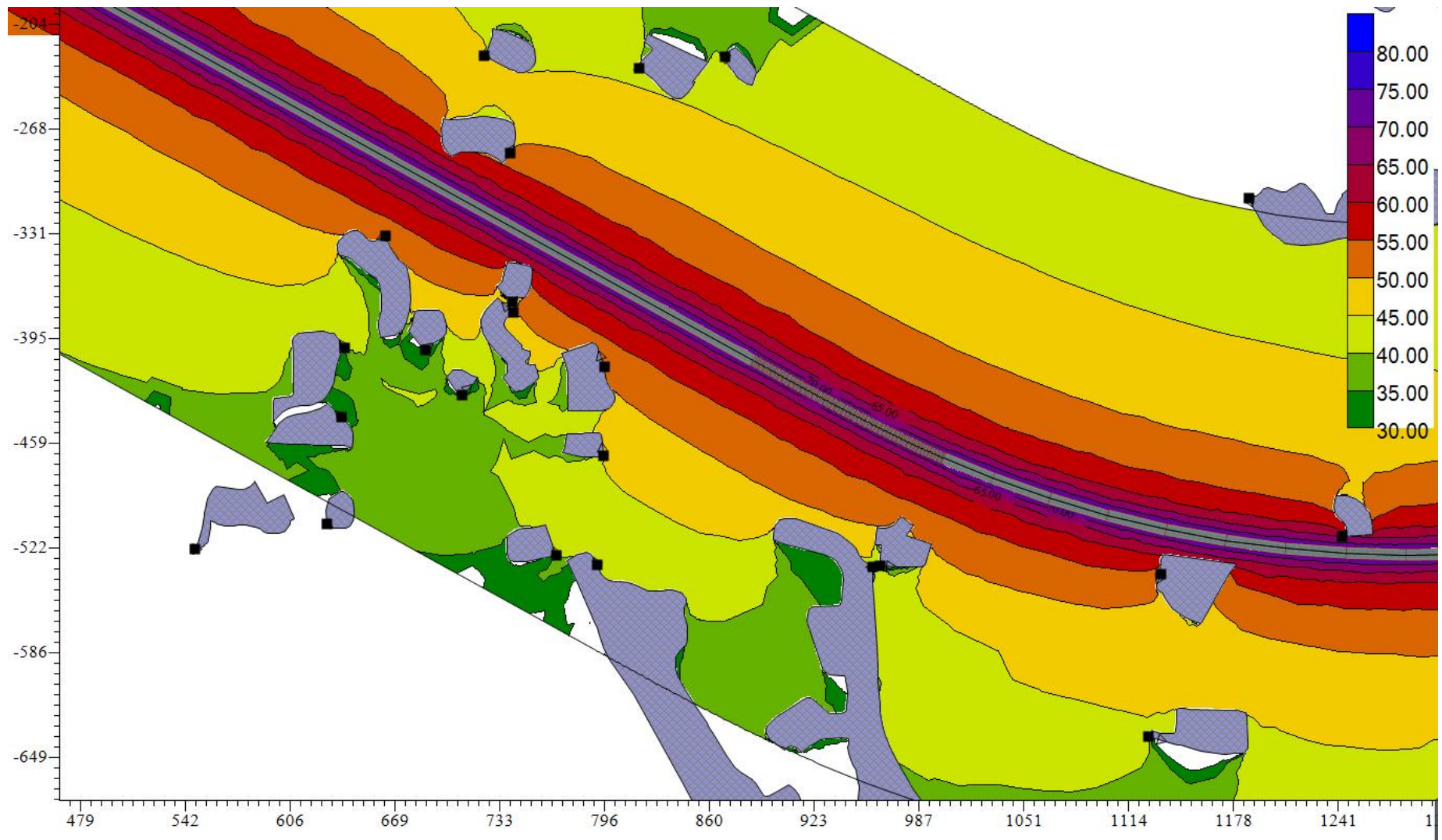
图 5.2-8.2 项目远期昼间交通噪声预测平面等声级线图（局部，居民分布较密集的路段 K2+000~K2+500）
