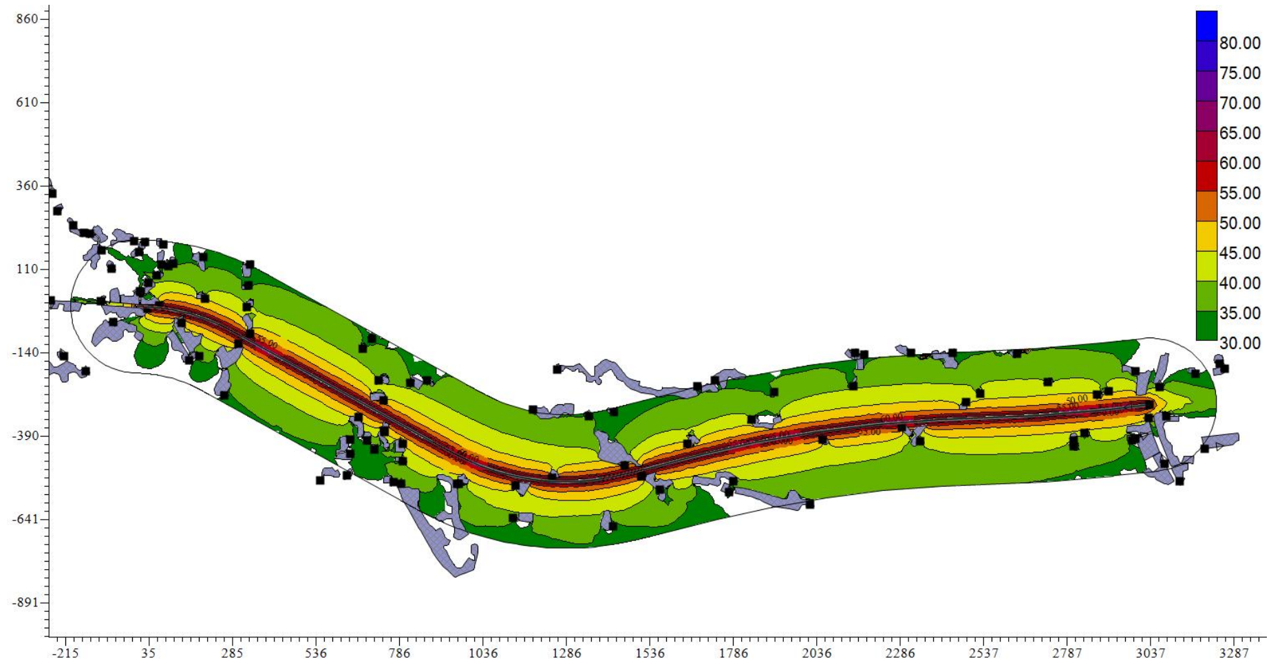
图 5.2-8.3 项目远期夜间交通噪声预测平面等声级线图（整体）
