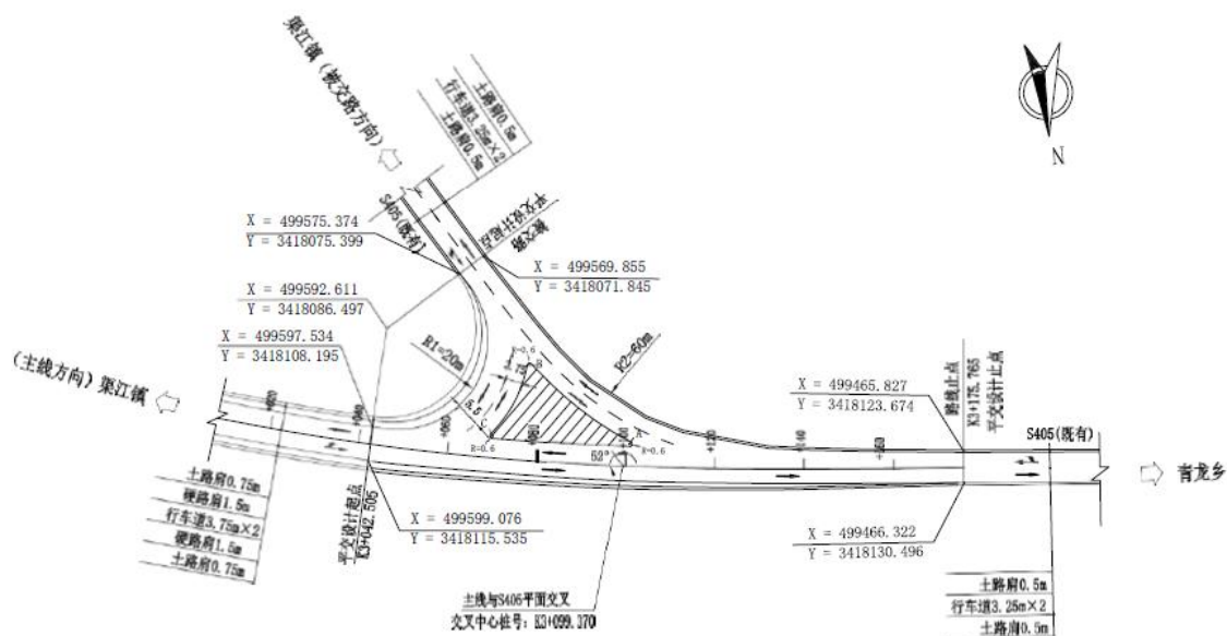
图 2.3-7 K3+009.370 平面交叉
