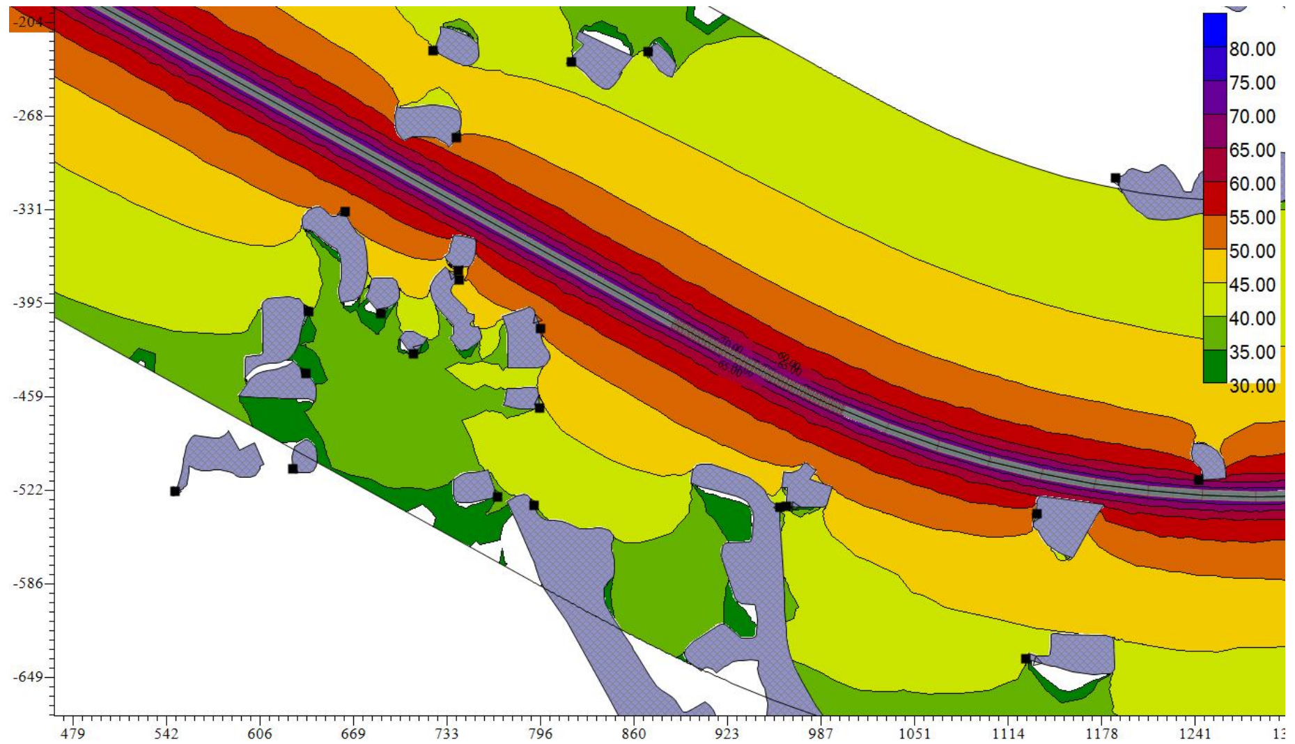
图 5.2-7.2 项目中期昼间交通噪声预测平面等声级线图（局部，居民分布较密集的路段 K2+000~K2+500）
