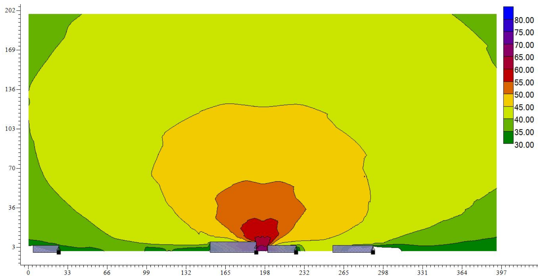
图 5.2-9.1 项目 K3+175.765 北侧 12m 农户处垂直等声值线图（近期昼间）
