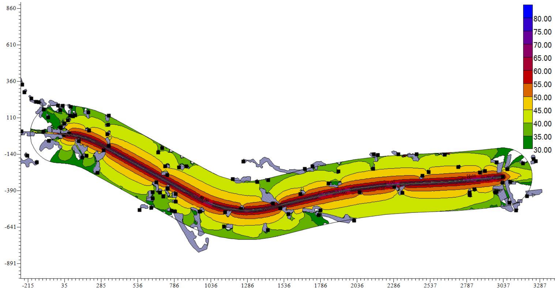
图 5.2-7.1 项目中期昼间交通噪声预测平面等声级线图（整体）
