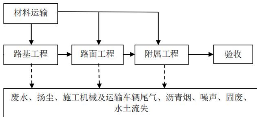
图 3.2-1 道路工程施工工艺流程及产污环节图
