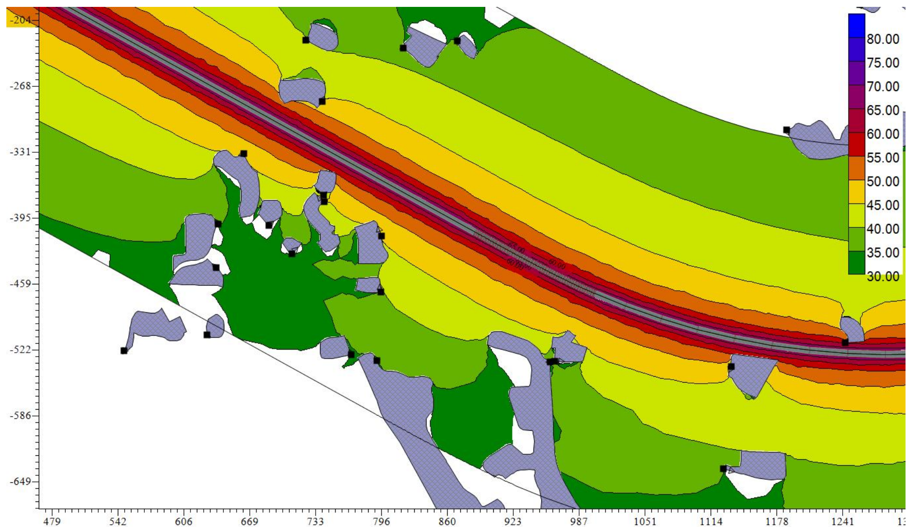
图 5.2-8.4 项目远期夜间交通噪声预测平面等声级线图（局部，居民分布较密集的路段 K2+000~K2+500）
