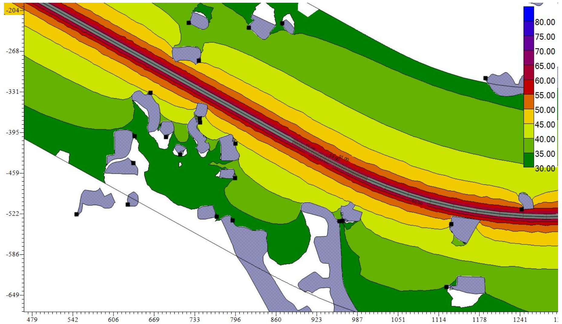
图 5.2-6.4 项目近期夜间交通噪声预测平面等声级线图（局部，居民分布较密集的路段 K2+000~K2+500）
