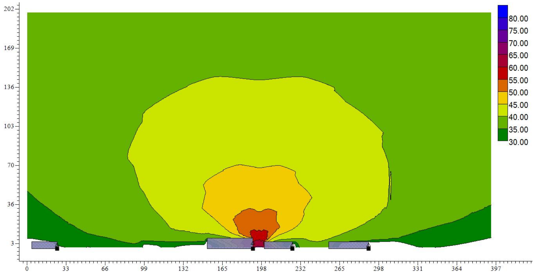
图 5.2-11.2 项目 K3+175.765 北侧 12m 农户处垂直等声值线图（远期夜间）
