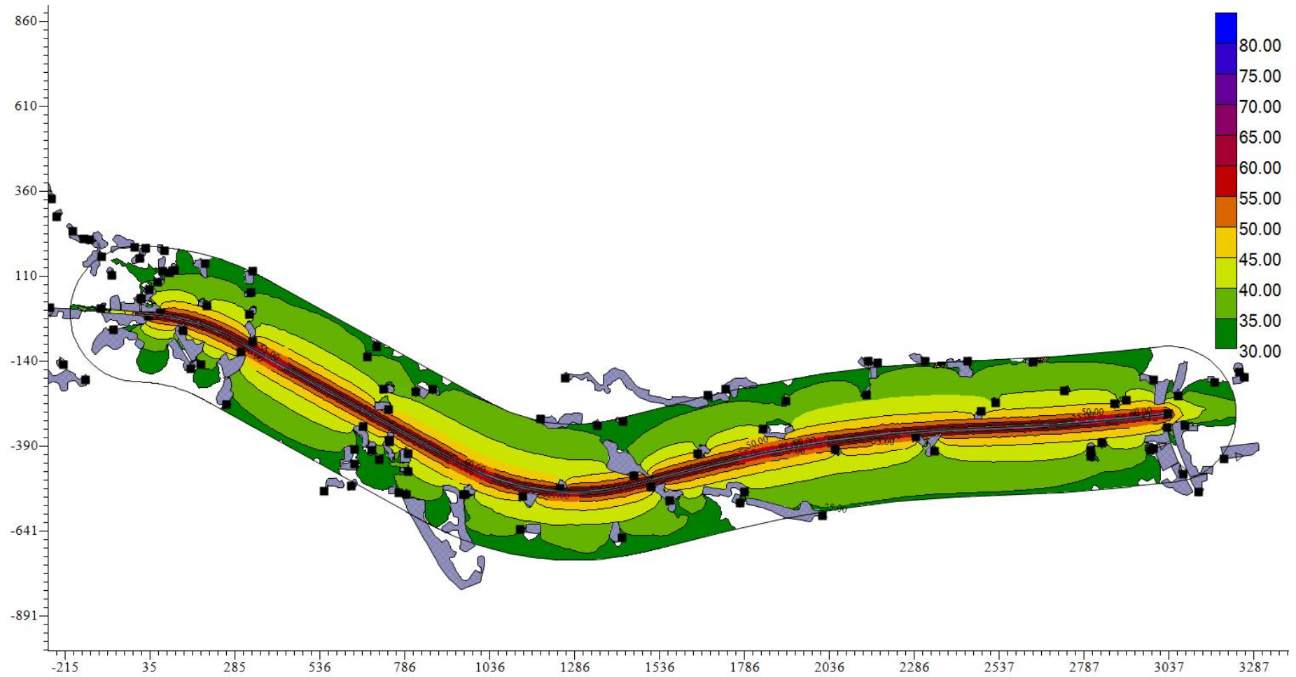
图 5.2-7.3 项目中期夜间交通噪声预测平面等声级线图（整体）
