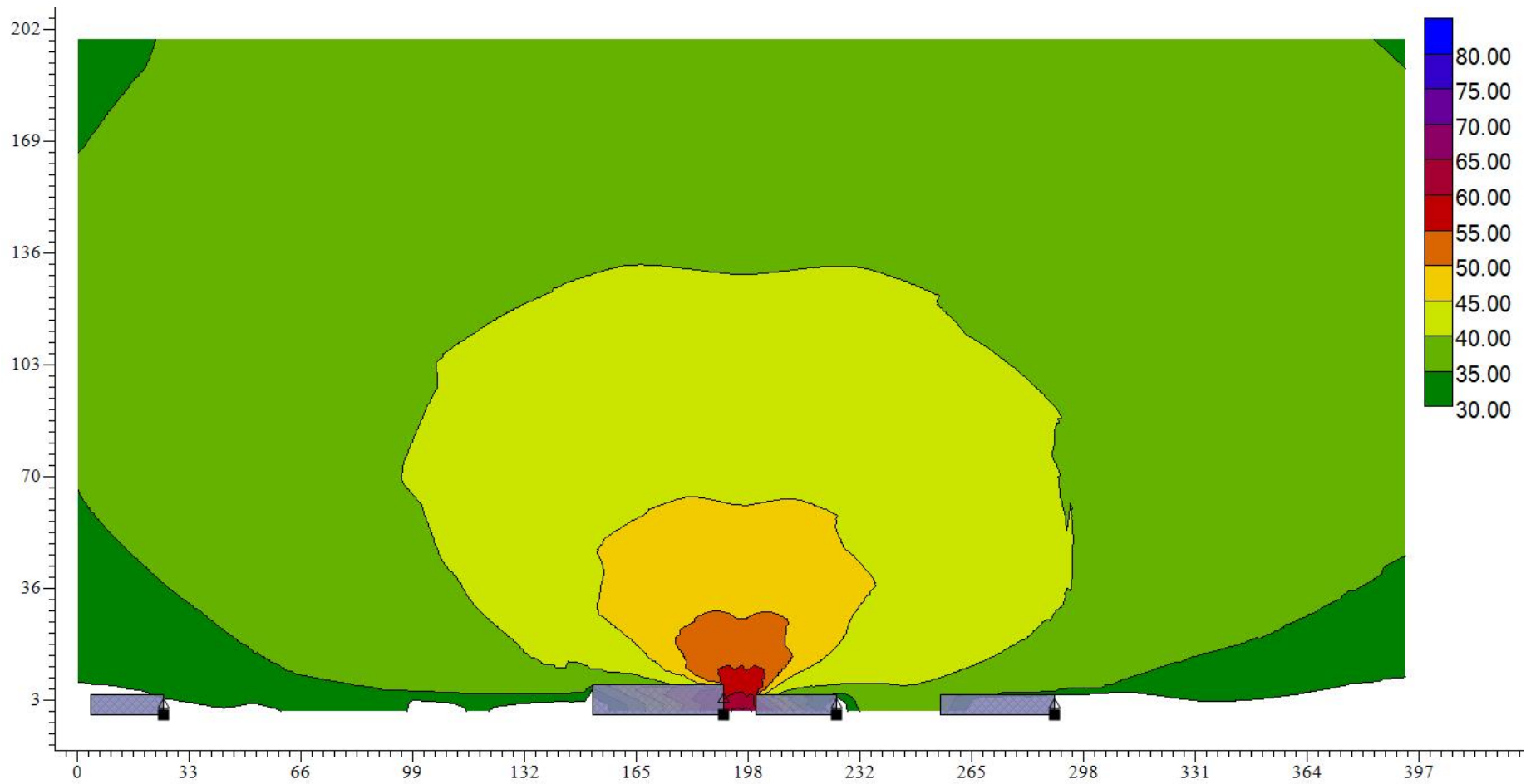
图 5.2-10.2 项目 K3+175.765 北侧 12m 农户处垂直等声值线图（中期夜间）
