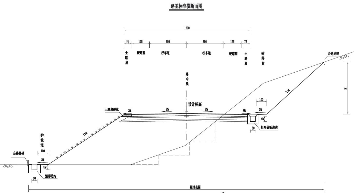
图 2.3-1 路基标准横断面图
