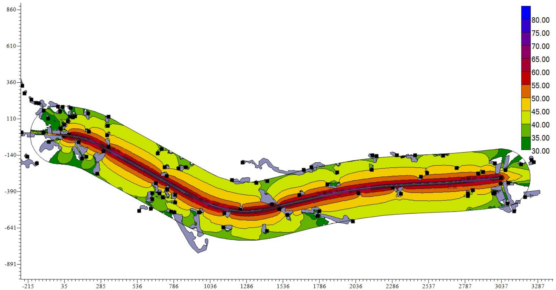
图 5.2-8.1 项目远期昼间交通噪声预测平面等声级线图（整体）
