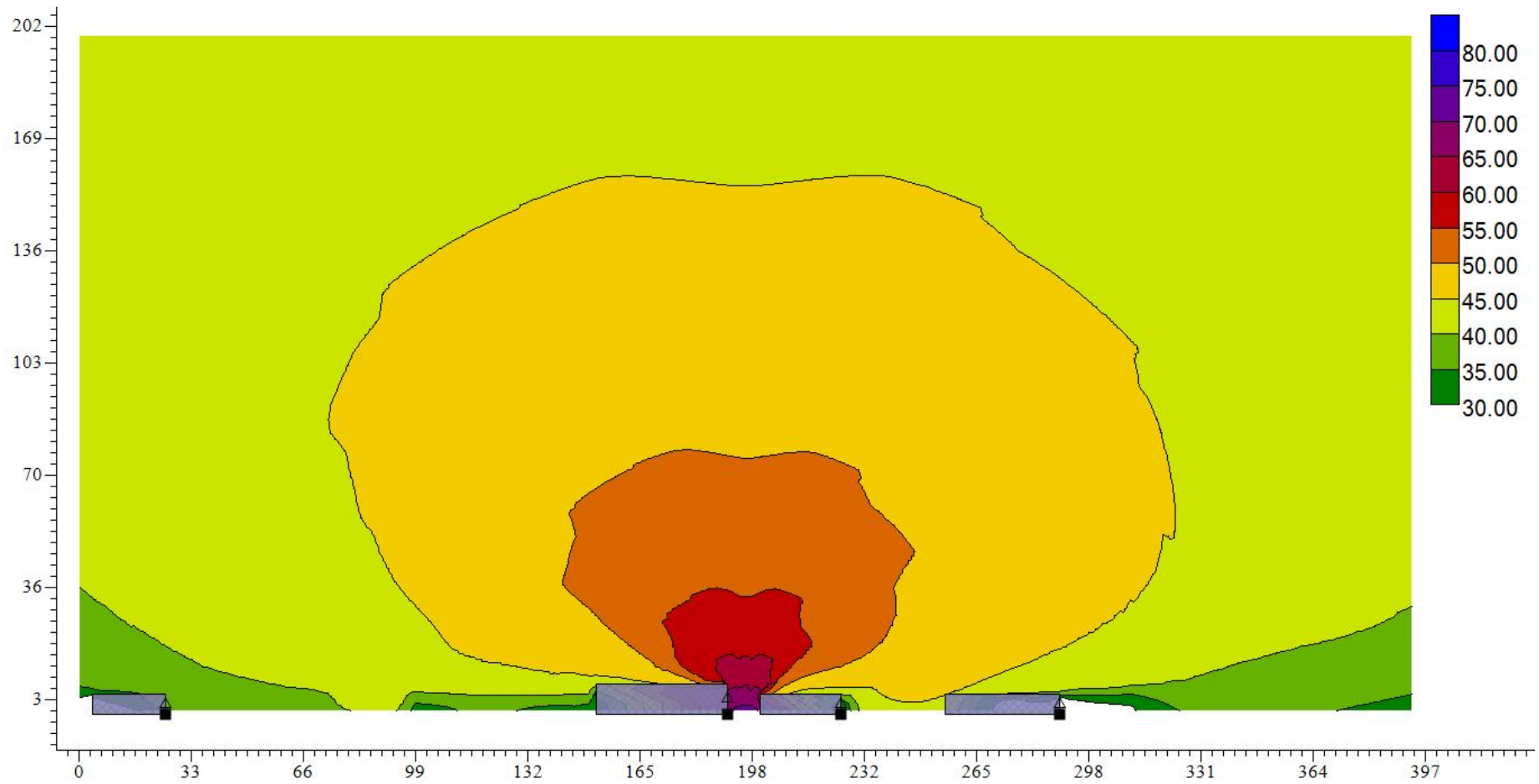
图 5.2-11.1 项目 K3+175.765 北侧 12m 农户处垂直等声值线图（远期昼间）
