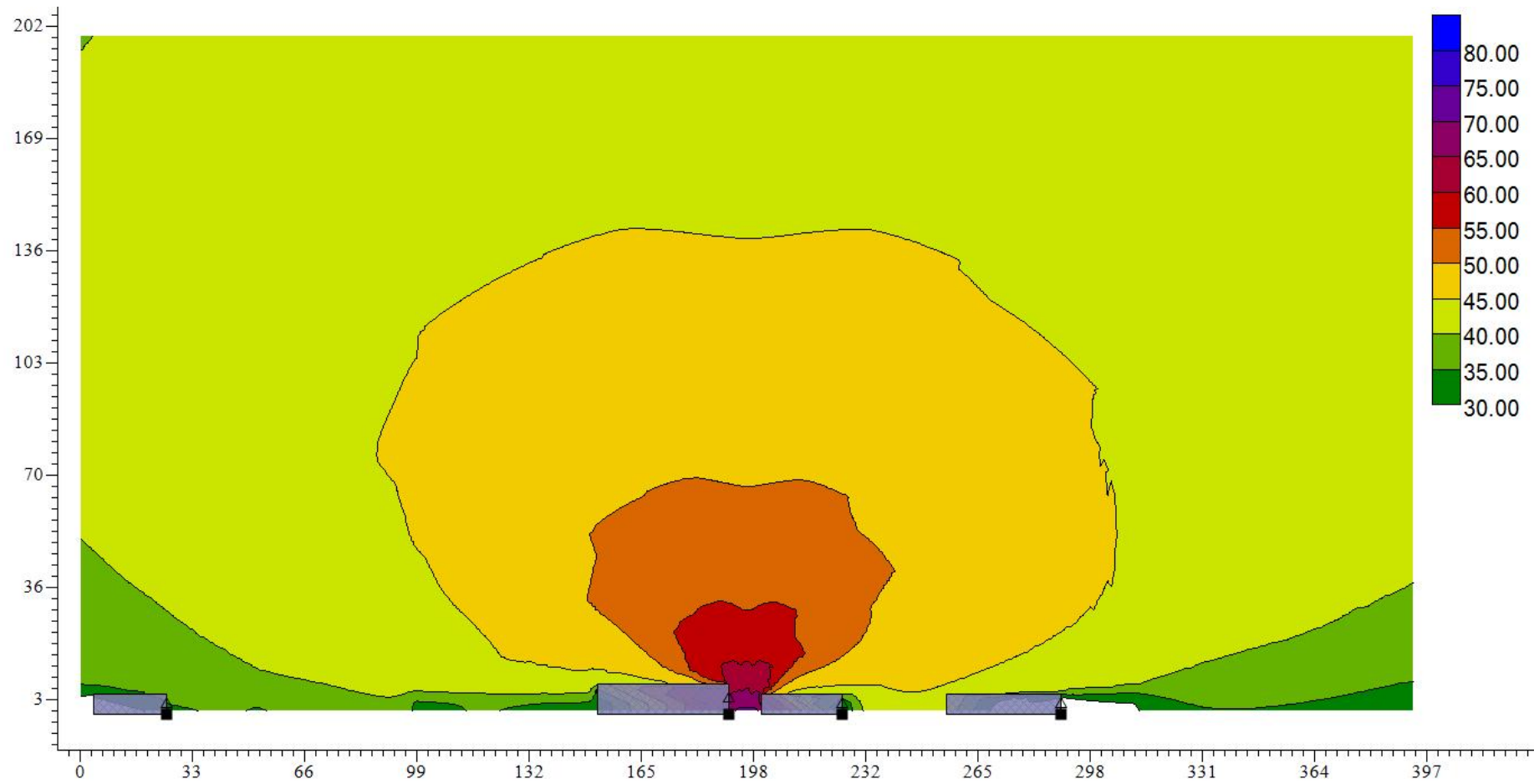
图 5.2-10.1 项目 K3+175.765 北侧 12m 农户处垂直等声值线图（中期昼间）
