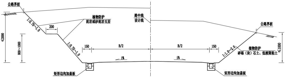
图 2.3-1 路基标准横断面图
