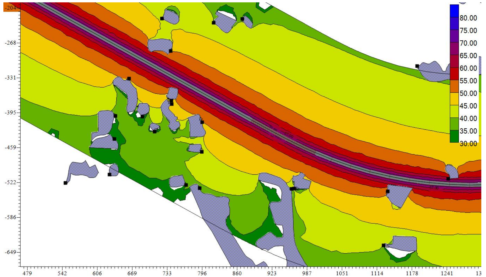
图 5.2-6.2 项目近期昼间交通噪声预测平面等声级线图（局部，居民分布较密集的路段 K2+000~K2+500）
