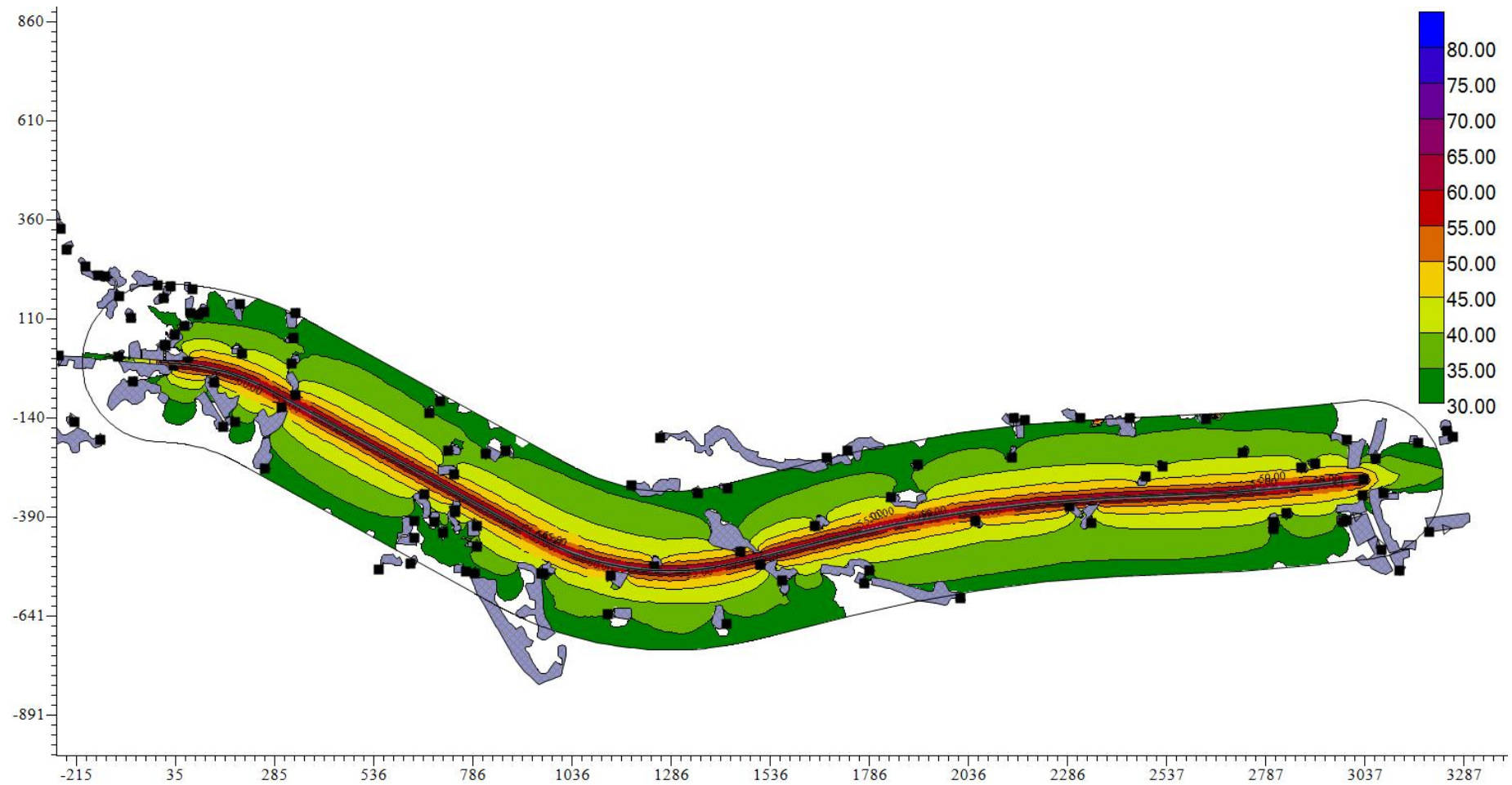
图 5.2-6.3 项目近期夜间交通噪声预测平面等声级线图（整体）
