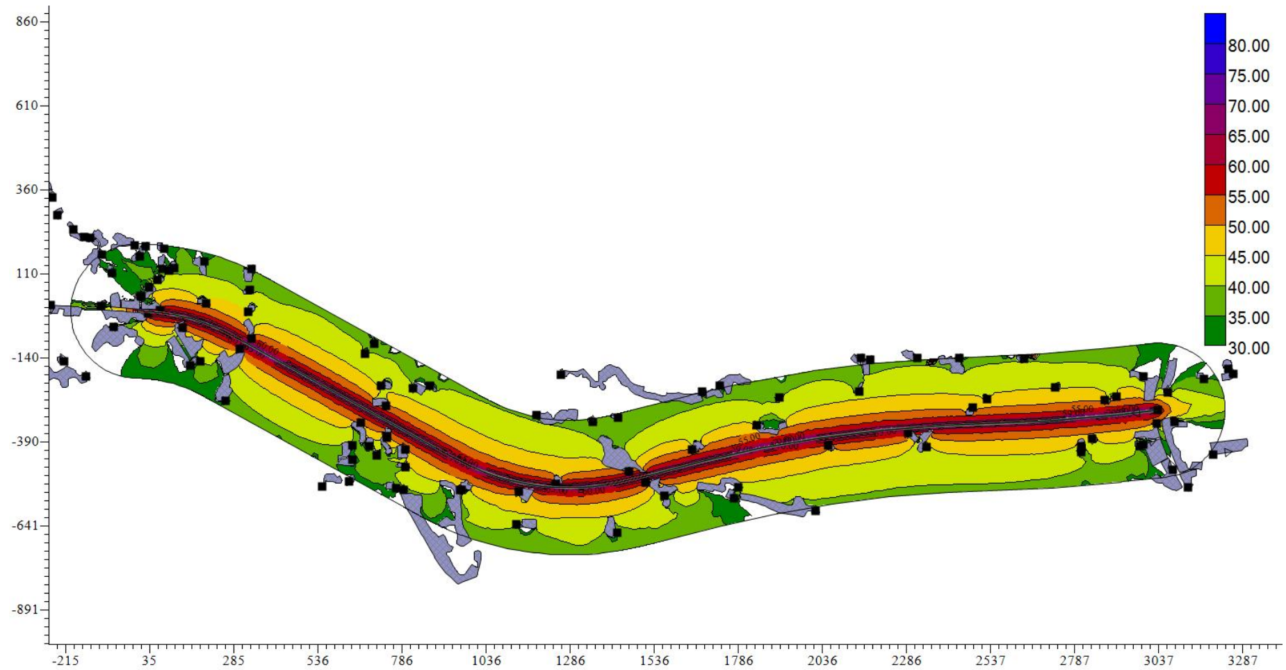
图 5.2-6.1 项目近期昼间交通噪声预测平面等声级线图（整体）
