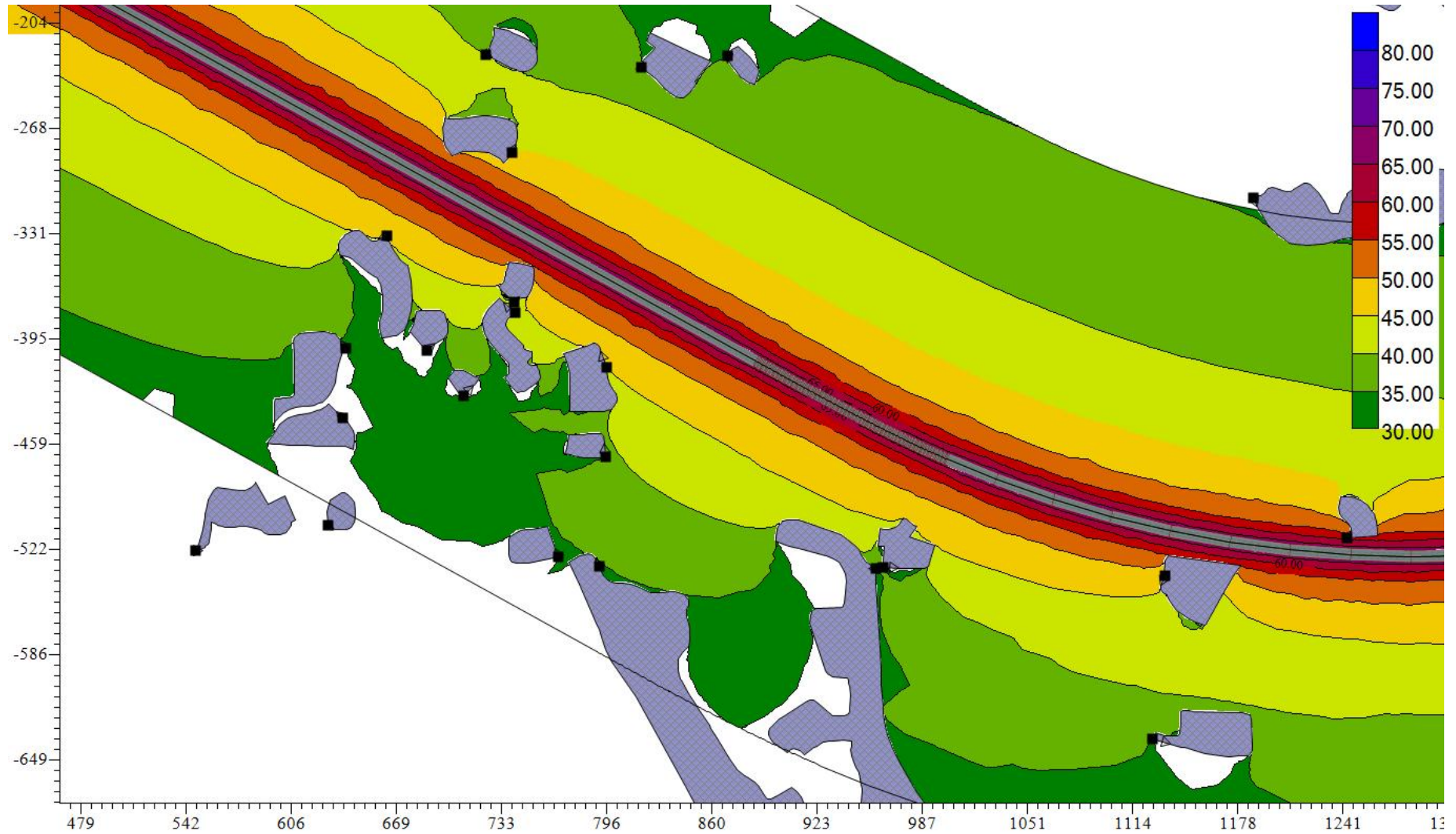
图 5.2-7.4 项目中期夜间交通噪声预测平面等声级线图（局部，居民分布较密集的路段 K2+000~K2+500）
