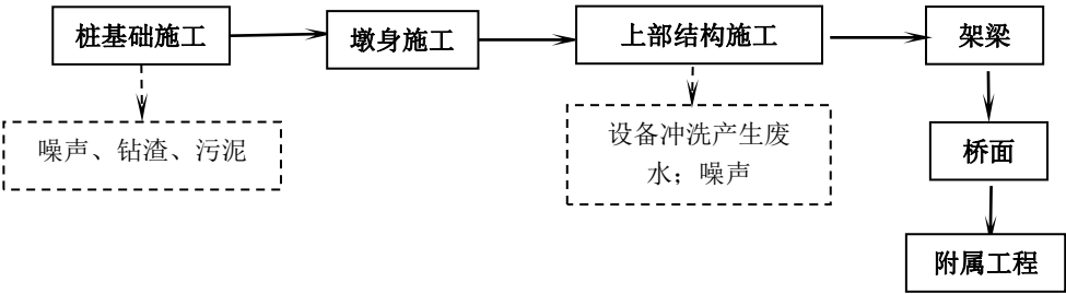
图 3.2-2 桥梁工程施工工艺流程及产污环节图
