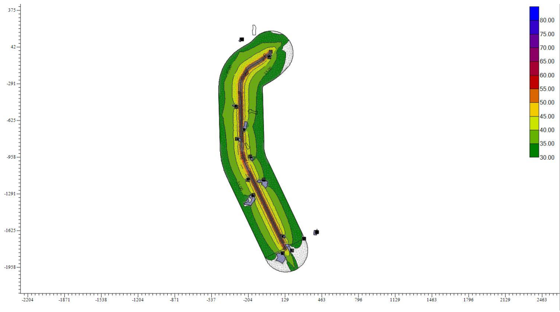
图 5.2-8 项目中期夜间交通噪声预测平面等声级线图
