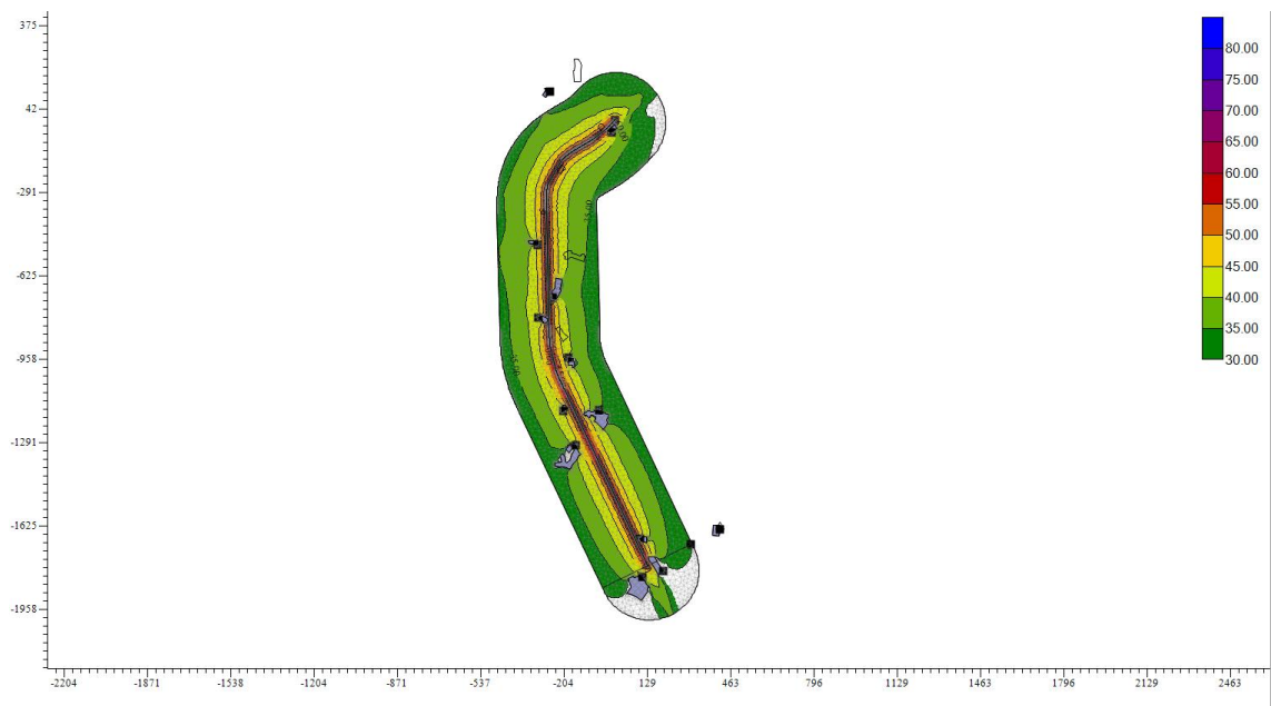
图 5.2-10 项目远期夜间交通噪声预测平面等声级线图
