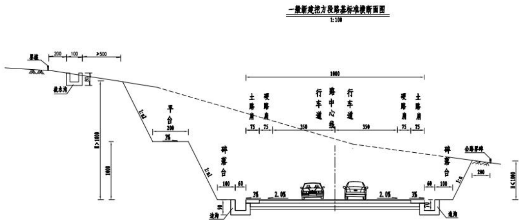
图 2.3-2 一般新建挖方段路基标准横断面图
