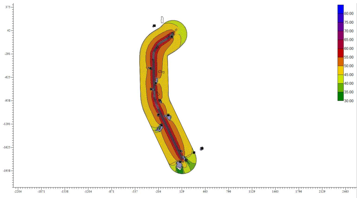
图 5.2-9 项目远期昼间交通噪声预测平面等声级线图
