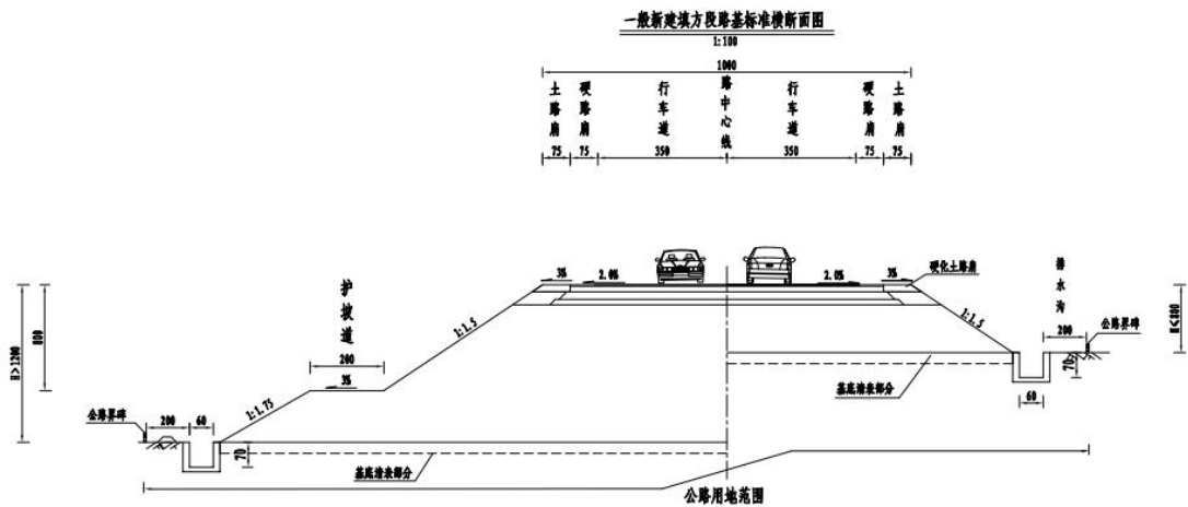
图 2.3-1 一般新建填方段路基标准横断面图
