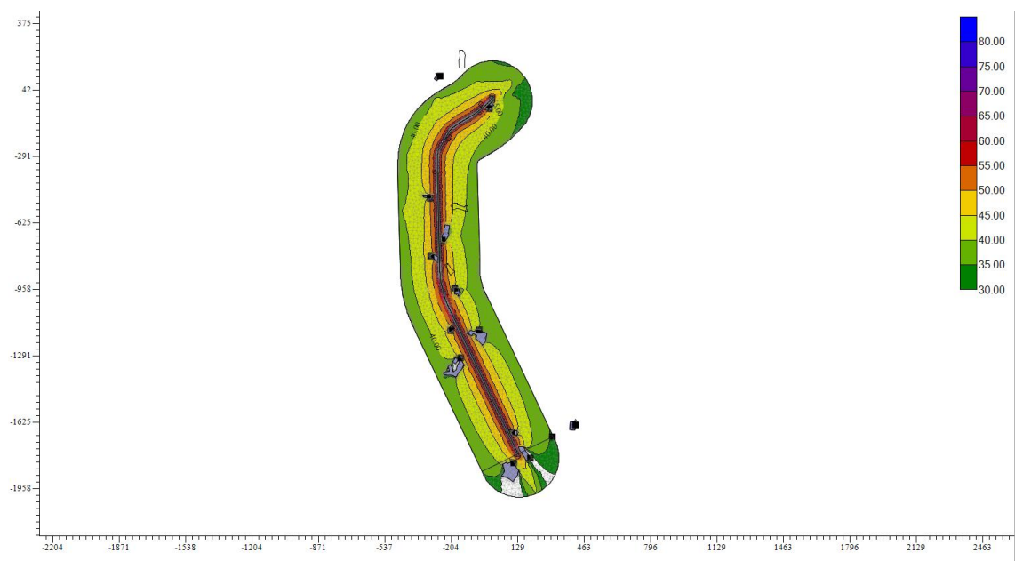
图 5.2-5 项目近期昼间交通噪声预测平面等声级线图
