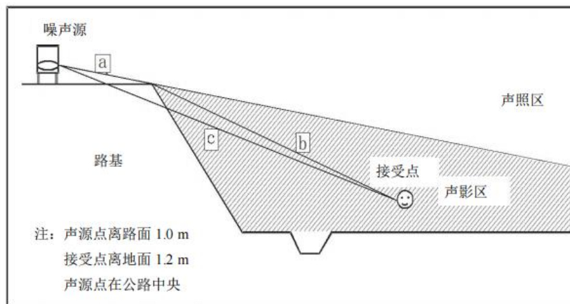
图 5.2-3 声程差 \delta 计算示意图
