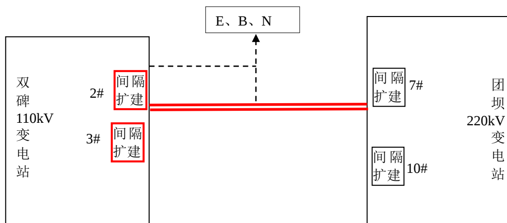
图 5-2 本项目运营期工艺流程及产污位置示意图
