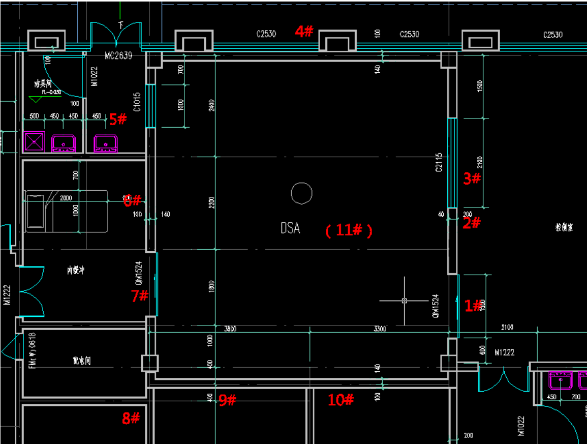
图11-1 介入治疗室评价点位图
